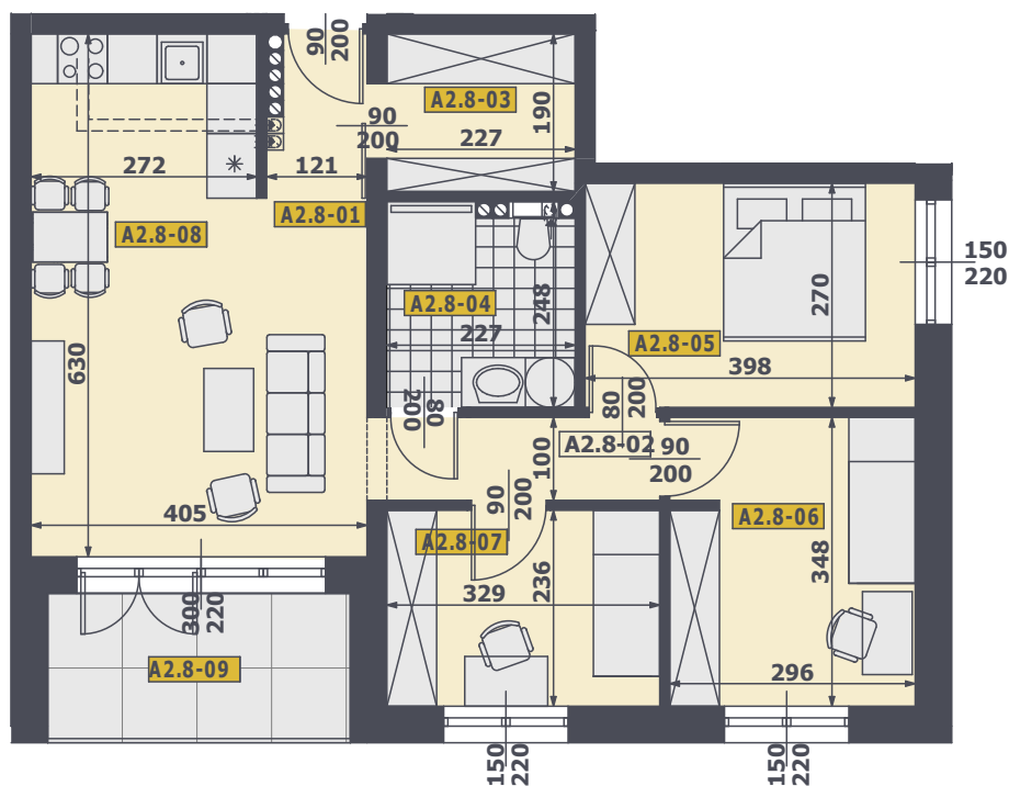
RZUT MIESZKANIA
