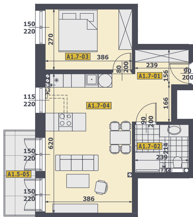
RZUT MIESZKANIA
