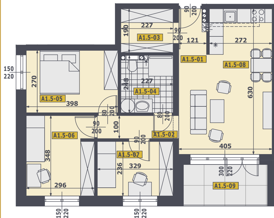
RZUT MIESZKANIA
