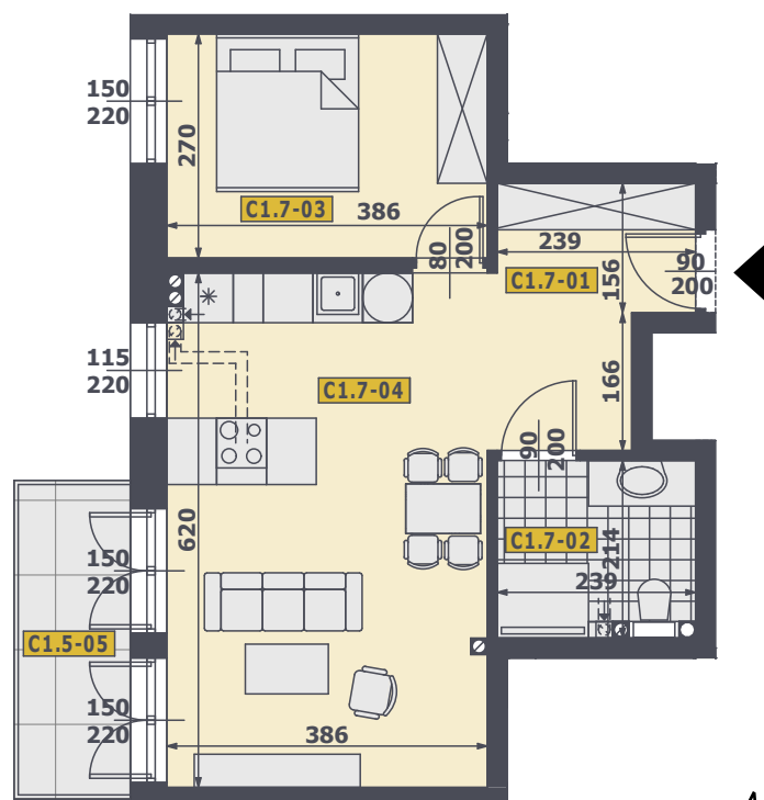
RZUT MIESZKANIA
