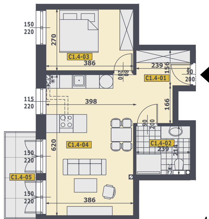
RZUT MIESZKANIA
