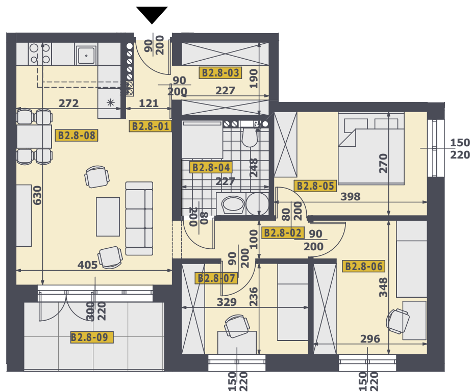
RZUT MIESZKANIA
